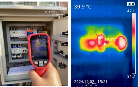
อุณหภูมิความร้อน 42.1°C
