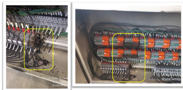
DC Panel Box No.3 ระเบิด
