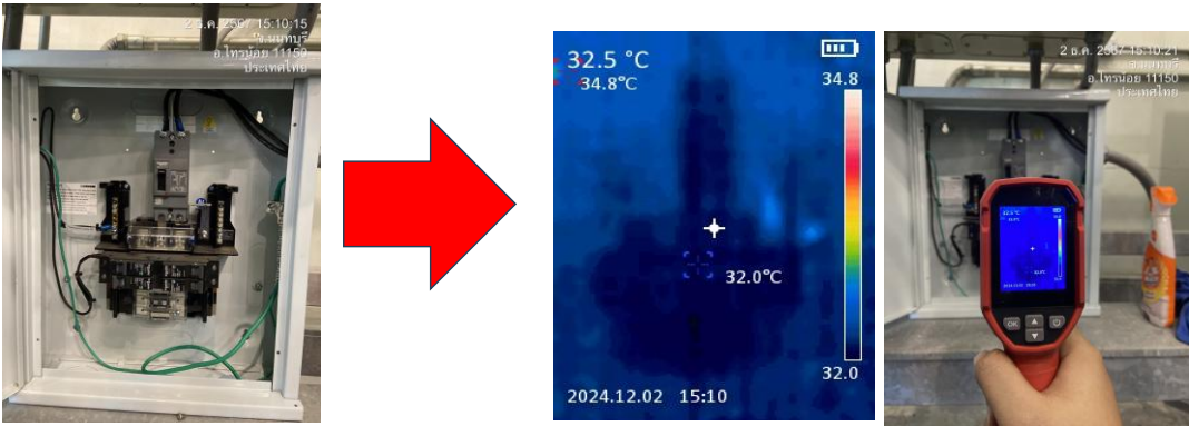
ภายในตู้ LP 32 °C
