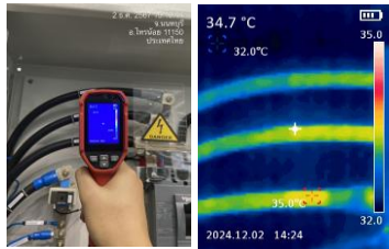
สาย MCCB 32 °C
