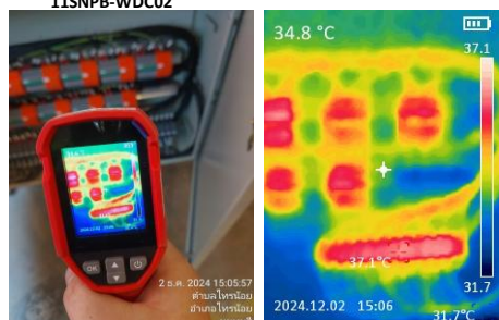
ภายในตู้ combination box อุณหภูมิ 37.1 °C
