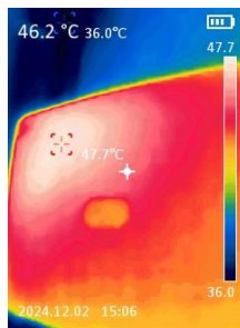
inverter No.4 อุณหภูมิ 47.7 °C
