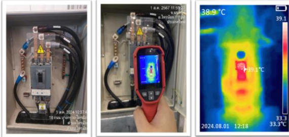
อุณหภูมิ MCCB Cabinet No.2 39.1 °C
